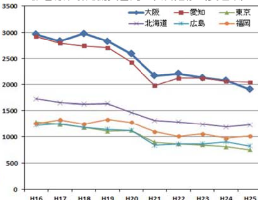
都道府県別死傷災害発生状況推移（製造業）
